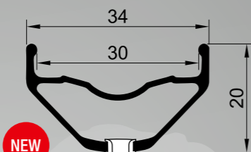
ENDURO PLUS - RX 2030 27,5" 532 g | 29" 567 g
