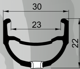
JUMBO - RX 2323 20" 480 g | 24" 610 g | 26" 710 g Extra pevný a odolný ráfek.
