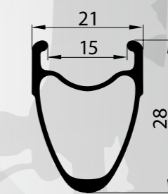
RAPID - RX 3515 622 x 15 545 g
