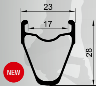
RX 4017 622 x 17 520 g
