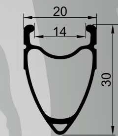
TAURUS - RX 5014 622 x 14 569 g
